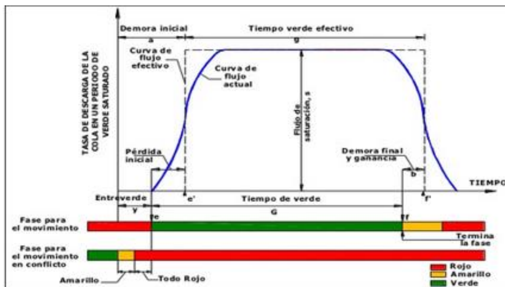
Figura 12: Modelo básico de flujo de saturación
