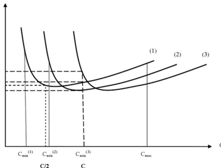
Figura 13: Comportamiento de la demora con el tiempo del ciclo
