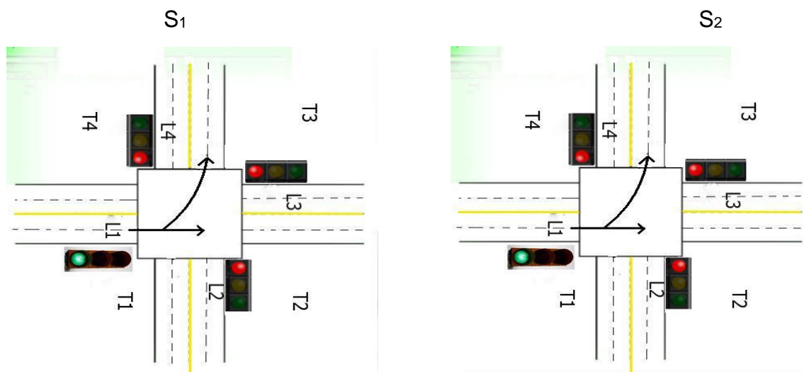
Figura 17: Existe coincidencia del tiempo verde en la fase dada.
