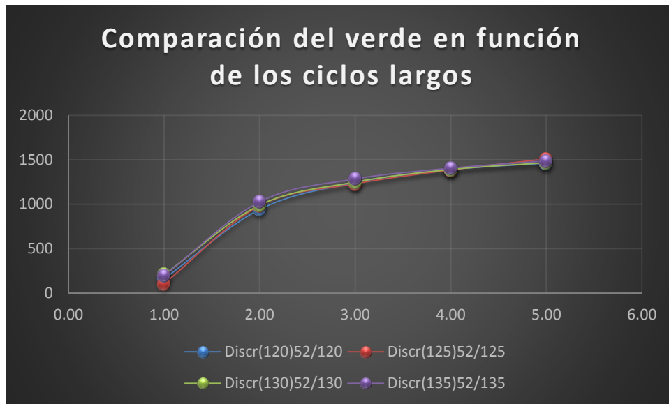
Figura 24: Comparación del verde efectivo y ciclo variable (Fuente: Tabla 6)
