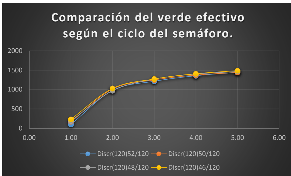
Figura 23: Comparación del verde efectivo con ciclo constante (Fuente: Tabla 5)
