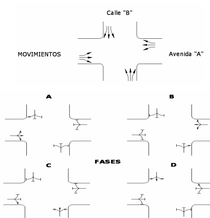
Figura 11: Fases en una intersección con semáforo
