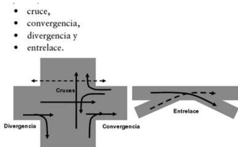
Figura 10: Conflictos en intersecciones
