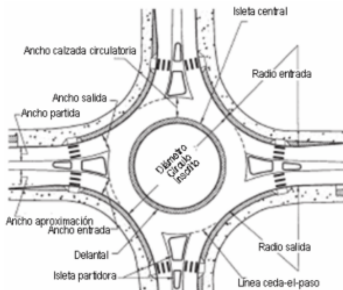
Figura 15: Elementos geométricos básicos de una rotonda
