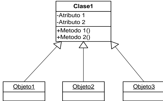
Figura 23. El símbolo de un diagrama de objeto. Tomado de: [Schmuller, 1999]
