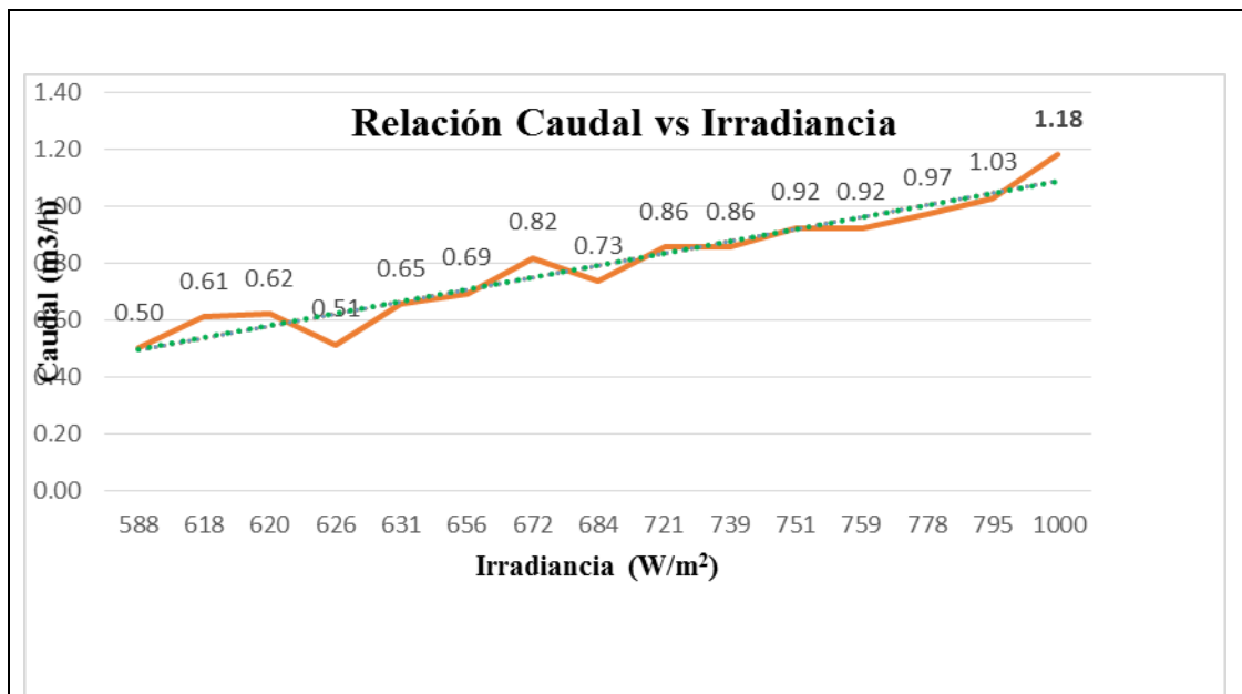
Gráfico No.4. Relación de caudal Vrs Irradiancia comunidad El Limón Estelí
