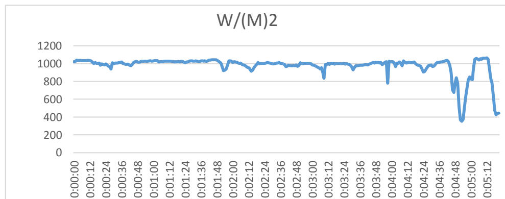
Gráfico No.5. Variación de la irradianción vrs tiempo comunidad El limón
