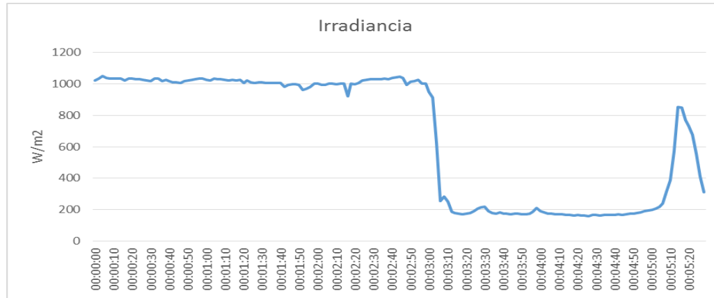
Gráfico No. 2- Valores de irradiación con Solarímetro PCE-SPM1
