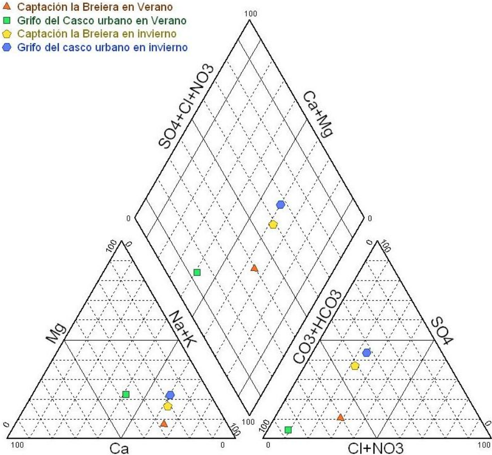
Figura 15. Diagrama de Piper tipo hidroquímico (HCO 3 – Ca) de muestras de agua por estación del año.
