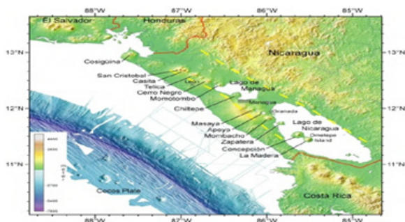
Mapa sobre las zonas de alta vulnerabilidad sísmica en nuestro país. Fuente: INETER
